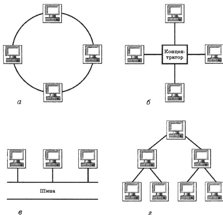
Рис. 4.15. Топологии локальных сетей: а — кольцевая, б — радиальная («звезда»), в — шинная, г — древовидная
